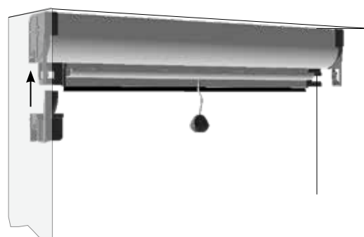
Posizione del cassonetto ormai fissato nel vano dai supporti per cassonetto alle contropiastre
