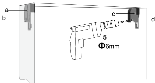
Posizione del cassonetto nelle contropiastre
