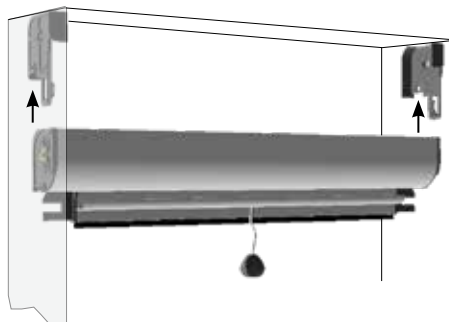
Far scorrere il supporto per cassonetto sx sulla contropiastre fino ad ottenere lo scatto di blocco
