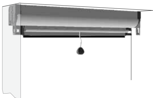
Far scorrere il supporto per cassonetto dx sulla contropiastre fino ad ottenere lo scatto di blocco
