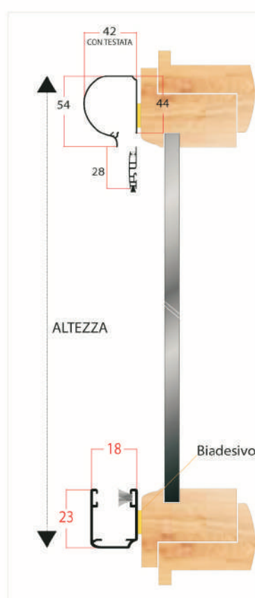
MONTAGGIO INFISSO FRONTALE CASS.42
