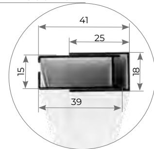
GUIDA TELESCOPICA
