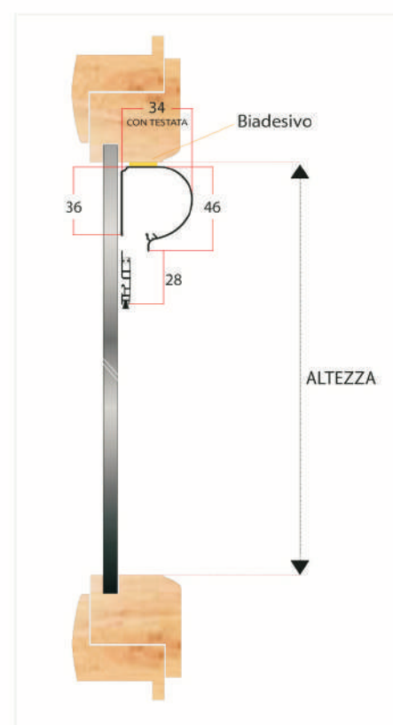
MONTAGGIO INTERNO FERMAVETRO CASS.34
