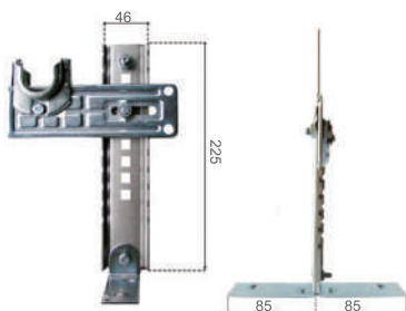
ACTA-96 Supporto a Bifora L=46 tipo Roma Euro 19,80 pz. (compreso 2 cuscinetti) Cod. 1088/R
