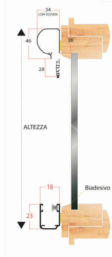
MONTAGGIO INFISSO FRONTALE CASS.34
