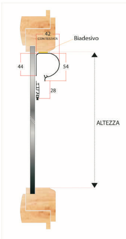
MONTAGGIO INTERNO FERMAVETRO CASS.42
